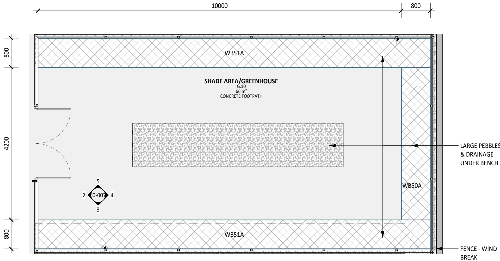
1 PLAN DETAIL 1 : 50
